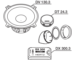
DSK 130.3
